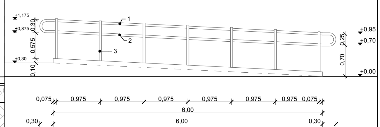
L1 nézet M=1:50
