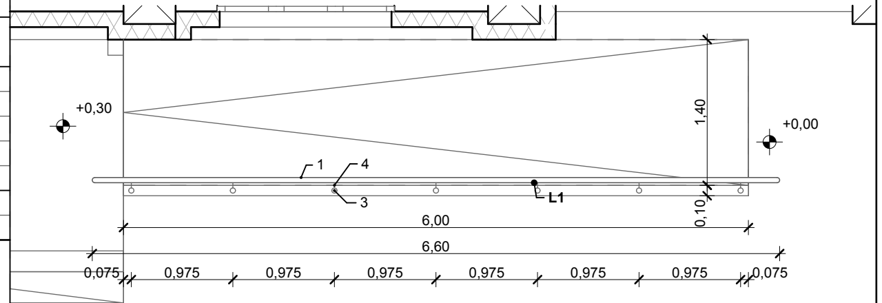
alaprjai nézet M=1:50
